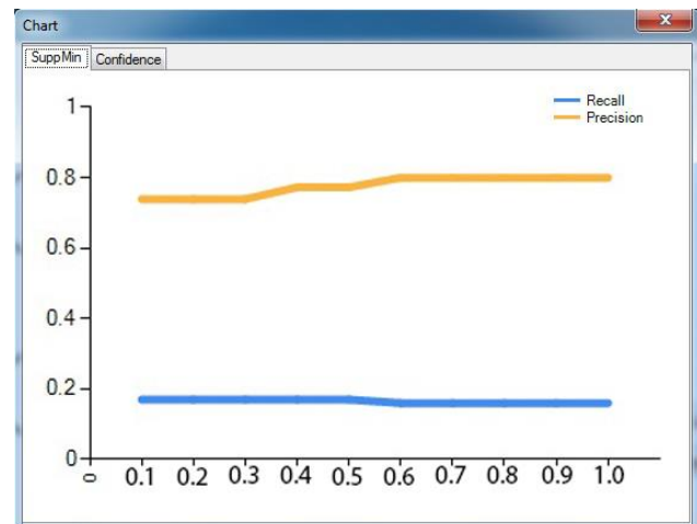
2a. \text{supp}_{\min}
