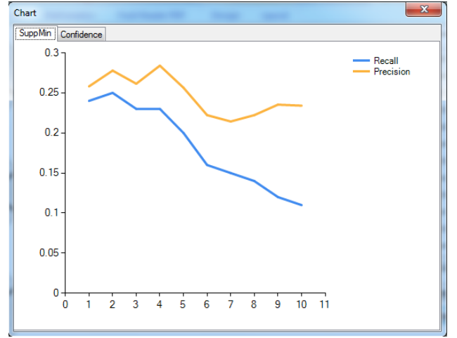
3a. supp_{min}
